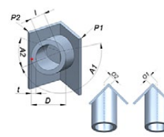
Rohr-Eckstoß
